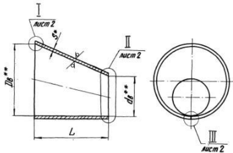
Переход сварной листовой эксцентрический
